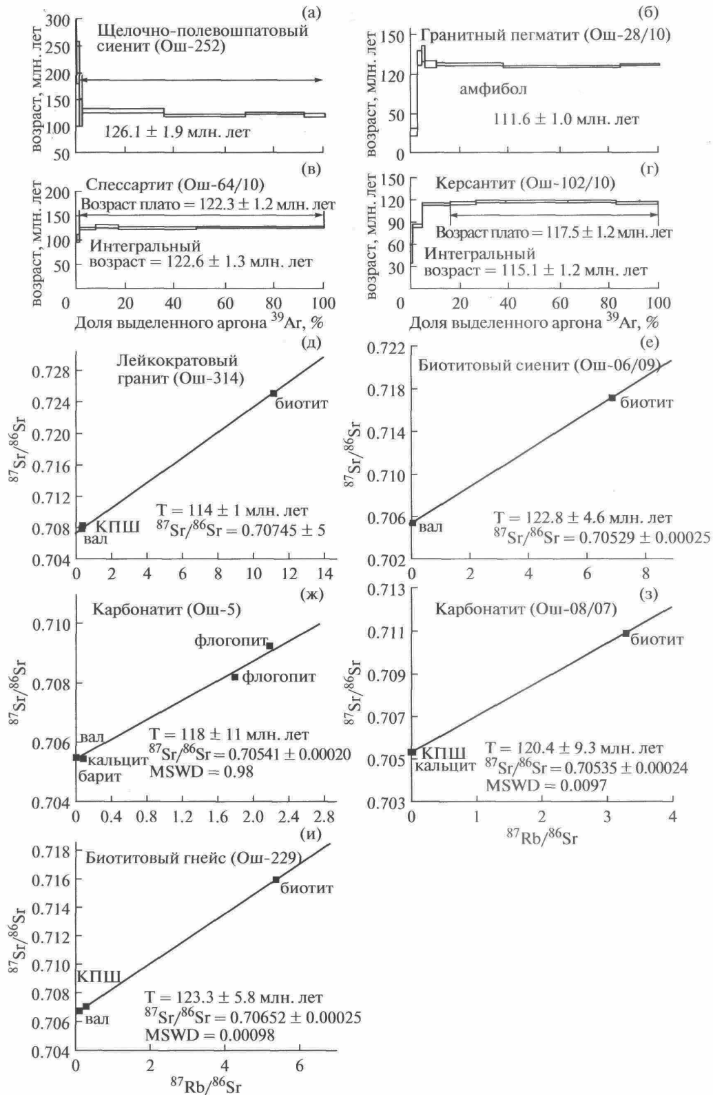
Рис. 5. ^{40}\text{Ar} - ^{39}\text{Ar} (а-г) возрастные спектры минералов и Rb-Sr (д-и) изохроны магматических и метаморфических пород на площади Ошурковского плутона.
