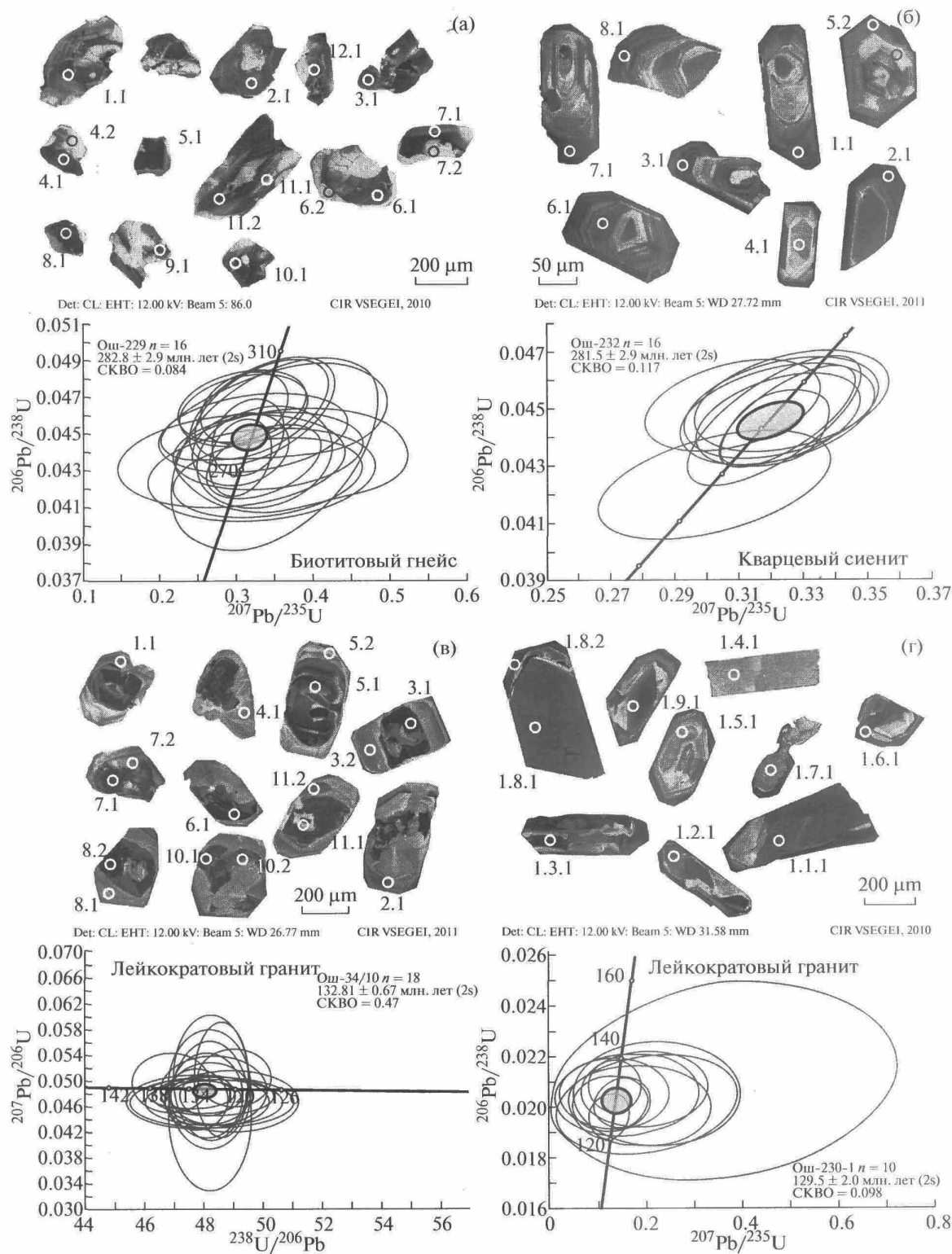
Рис. 4. Диаграммы с конкордией для цирконов Ошурковского плутона и вмещающих пород:
