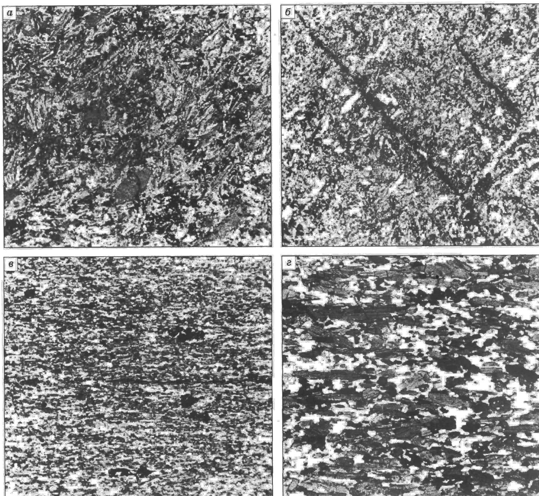
Рис. 4. Структуры метавулканитов.
