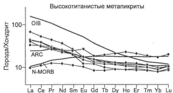
Рис. 10. Диаграммы концентраций редкоземельных элементов, нормированные к хондриту [Sun, McDonough, 1989], для метавулканитов Тункинского террейна.
