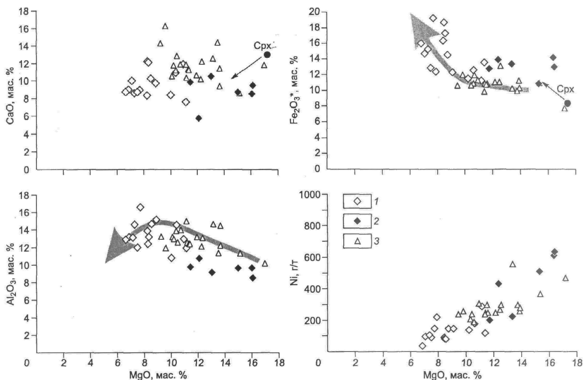
Рис. 8. Вариации содержаний CaO, Al 2 O 3 , Fe 2 O 3 и Ni в зависимости от MgO в метавулканитах Тункинского террейна.
