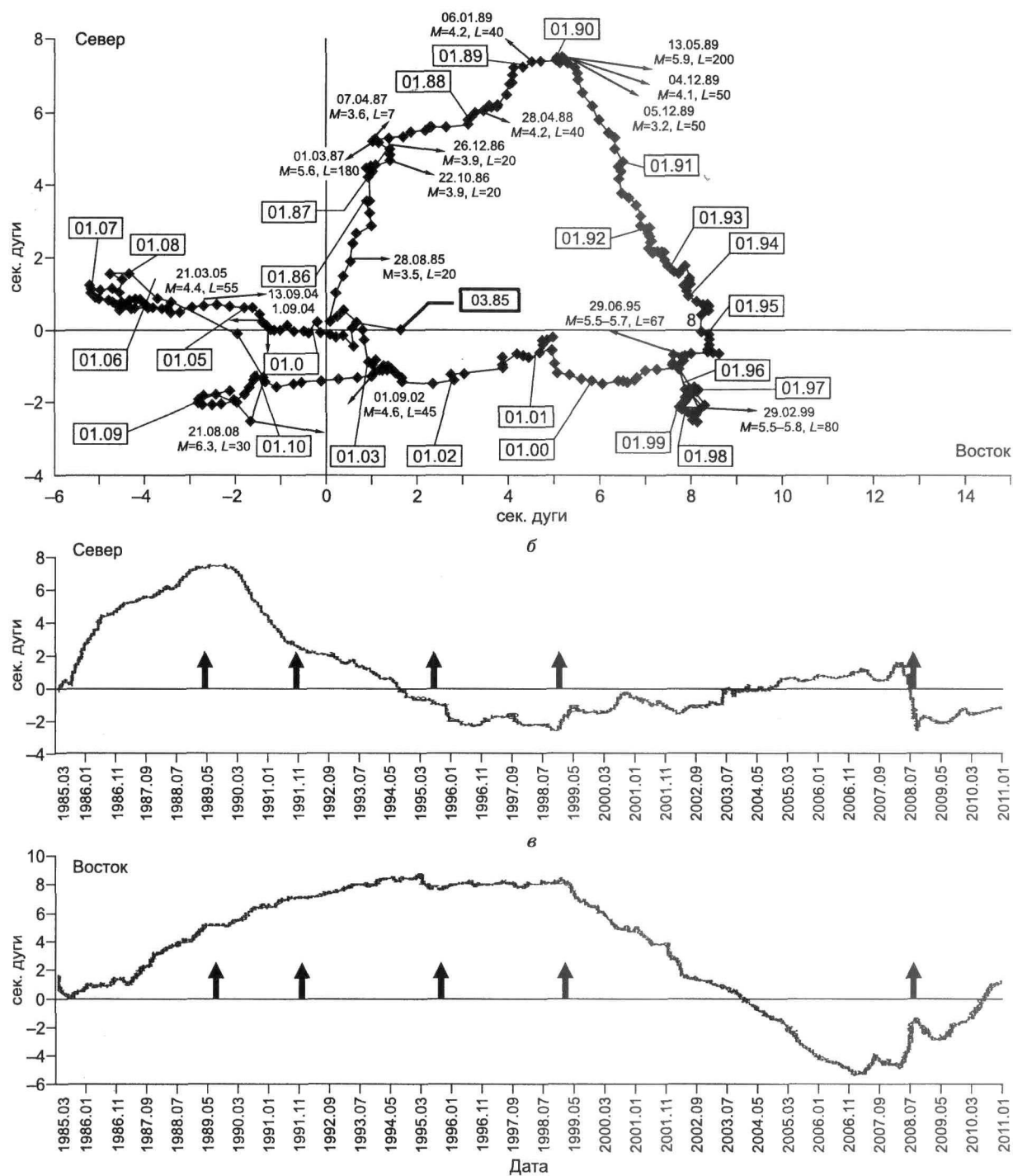
Рис. 1. Записи хода наклона в штольне станции Талая.
