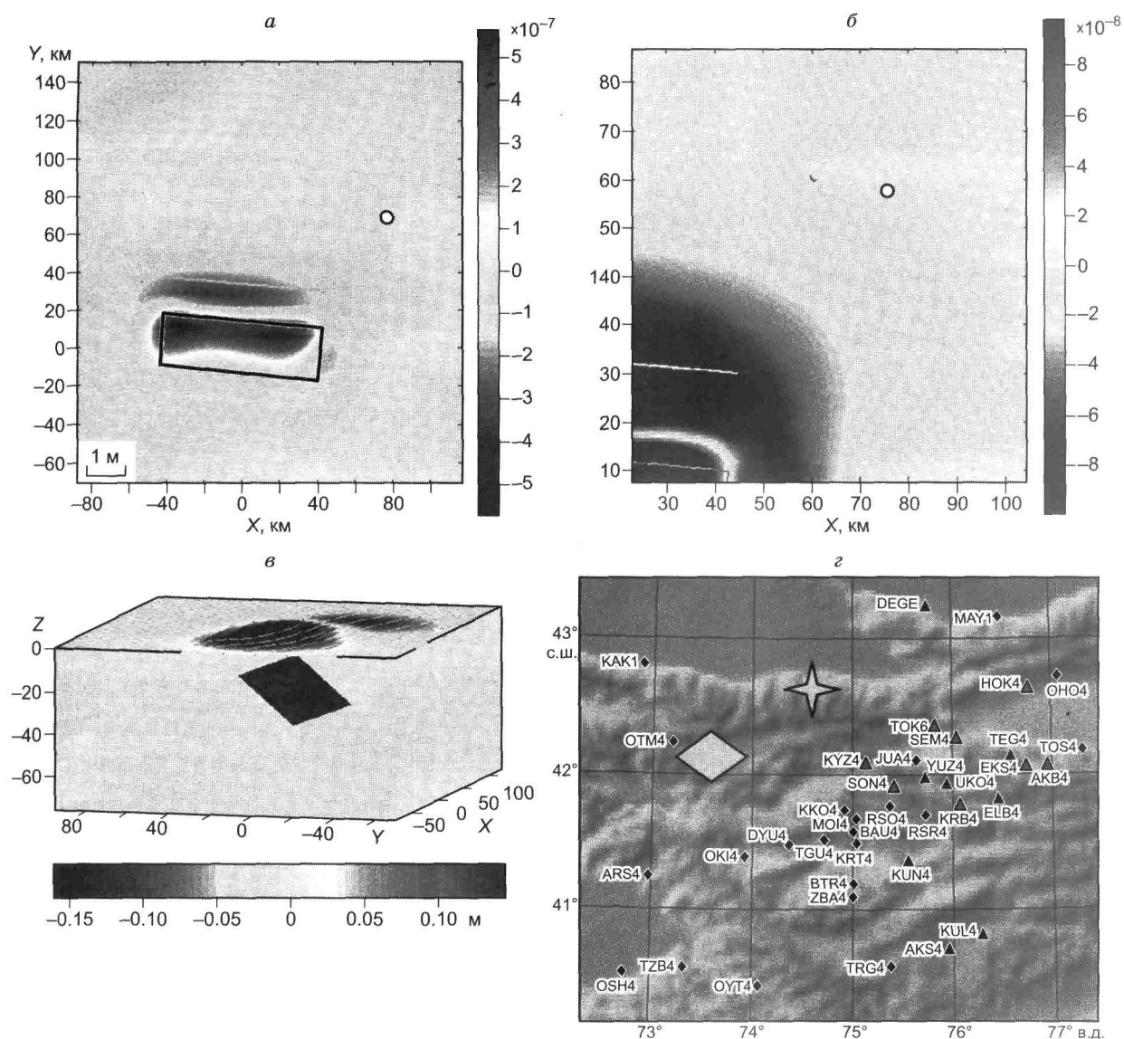
Рис. 4. Моделирование деформаций при Суусамырском землетрясении.
