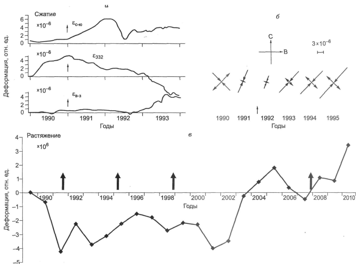
Рис. 2. Вариации деформации на станции Талая.
