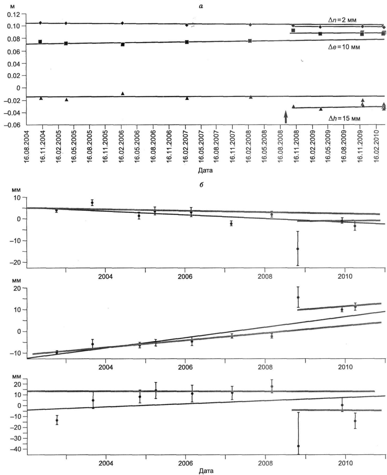
Рис. 10. Экспериментальные данные по смещениям при Култукском землетрясении.
