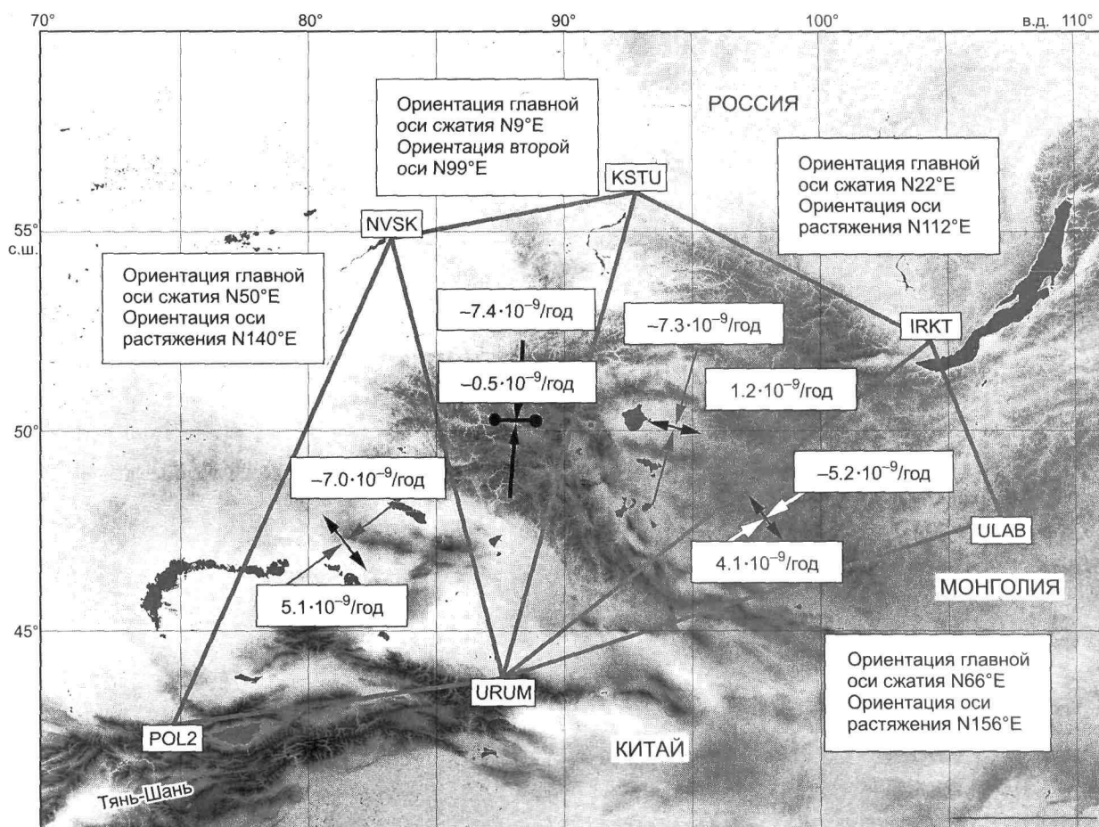
Рис. 5. Результаты определения скоростей деформаций.
