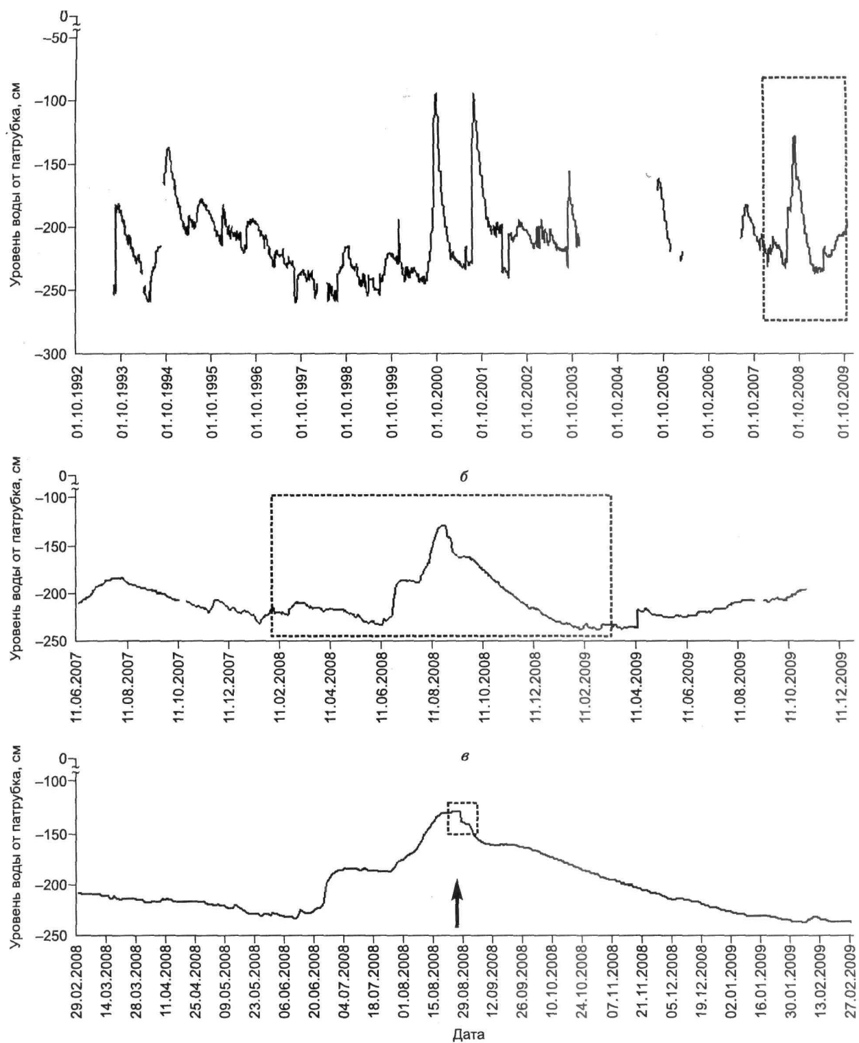
Рис. 6. Запись водного уровня в скважине Талая на разных периодах.
