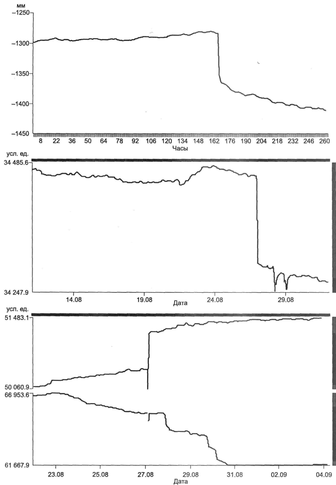
Рис. 7. Косейсмические изменения деформации на станции Талая, по результатам измерений разными видами датчиков.
