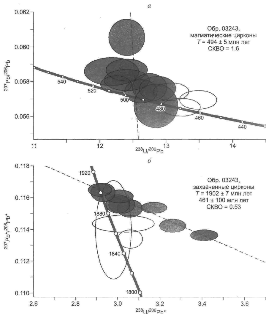
Рис. 8. Диаграммы ^{207}\text{Pb}/^{206}\text{Pb} — ^{238}\text{U}/^{206}\text{Pb} (а) и ^{207}\text{Pb}^*/^{206}\text{Pb}^* — ^{238}\text{U}/^{206}\text{Pb}^* (б) [Tera, Wasserburg, 1972] для цирконов из гибридных пород (обр. 03243).
