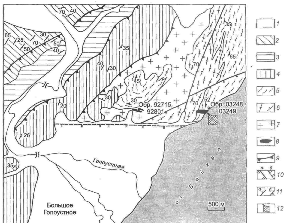
Рис. 2. Схема геологического строения района распространения раннепалеозойских долеритов (пос. Большое Голоустное).
