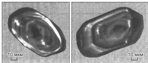
Рис. 7. Катодолюминесцентные изображения кристаллов циркона первой группы (обр. 03243).
