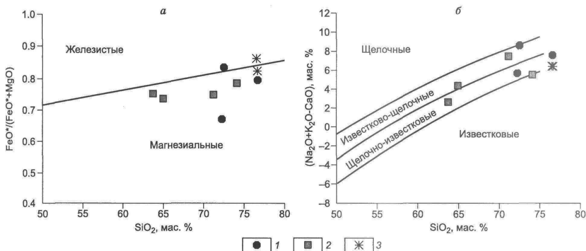
Рис. 5. Диаграммы \text{FeO}^*/(\text{FeO}^* + \text{MgO}) — \text{SiO}_2 (а), \text{Na}_2\text{O} + \text{K}_2\text{O} - \text{CaO} — \text{SiO}_2 (б) [Frost et al., 2001] для лейкогранитов (1), гибридных пород крупной дайки (2) и мигматизированных гнейсов (3) Голоуспенского выступа фундамента Сибирского кратона.
