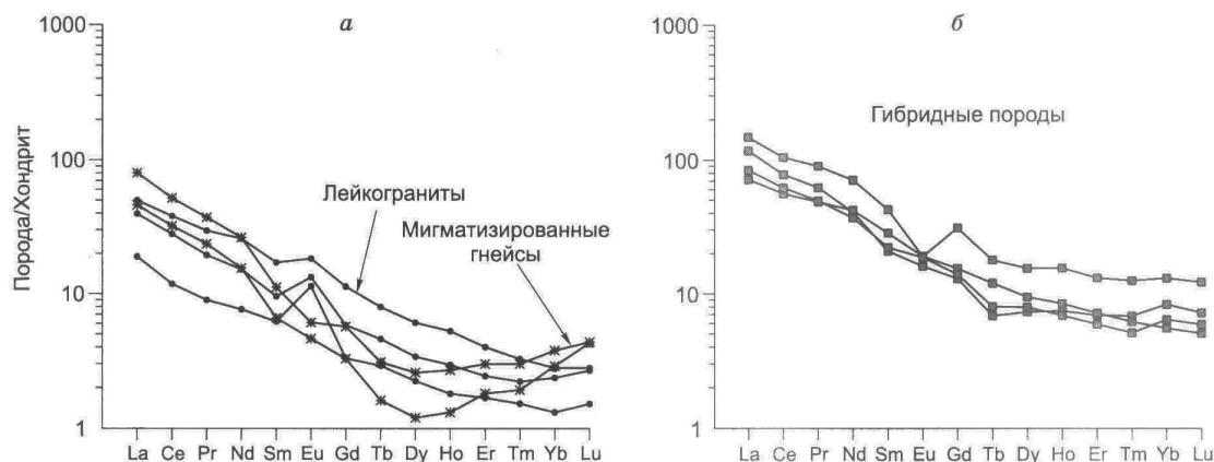
Рис. 6. Спектры распределения редкоземельных элементов, нормализованные к хондриту [Накамура, 1974], для лейкогранитов из обособлений в эндоконтактовой зоне крупной дайки долеритов, и палеопротерозойских мигматизированных гнейсов (а), а также гибридных пород крупной дайки (б).
