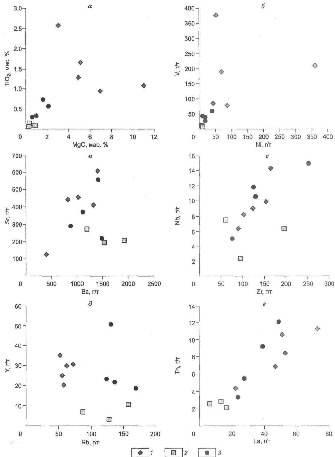
Рис. 9. Диаграммы \text{TiO}_2 — \text{MgO} (a), \text{V} — \text{Ni} (б), \text{Sr} — \text{Ba} (в), \text{Nb} — \text{Zr} (г), \text{Y} — \text{Rb} (д), \text{Th} — \text{La} (е) для долеритов даек Голоуспенского выступа (1), лейкогранитов из обособлений в эндоконтактовой зоне крупной дайки долеритов (2) и гибридных пород крупной дайки (3).
