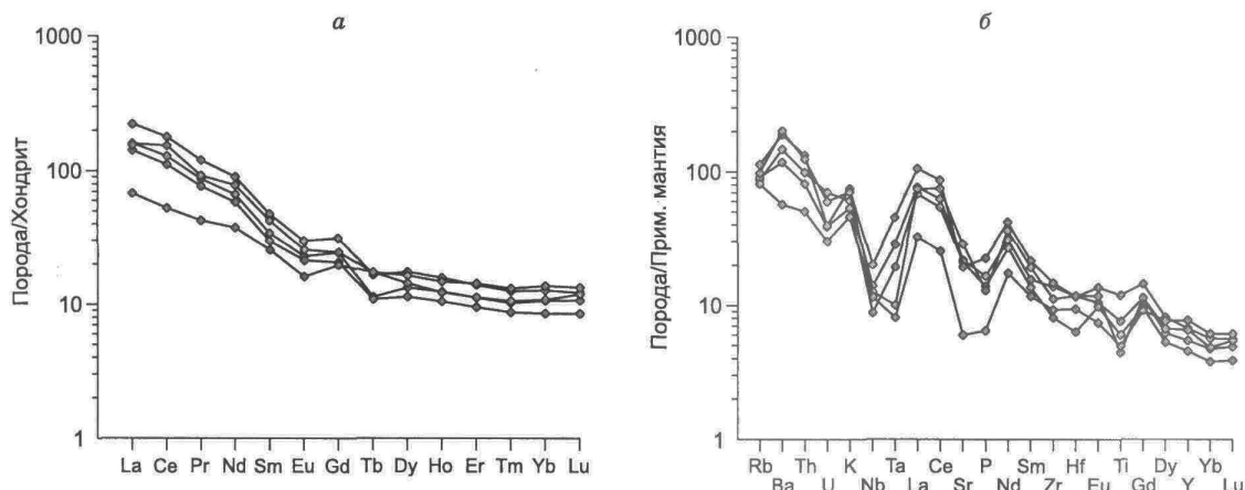
Рис. 4. Спектры распределения редкоземельных элементов, нормализованные к хондриту [Nakamura, 1974] (а), и мультиэлементные спектры, нормализованные к примитивной мантии [Sun, McDonough, 1989] (б), для долеритов даек Голоуспенского выступа.
