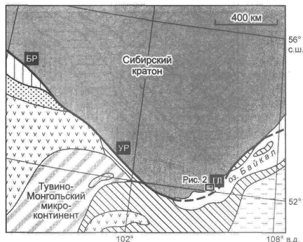
Рис. 1. Схема основных тектонических структур Южной Сибири (модифицировано по [Волкова, Складьев, 2007; Ножкин, 2009]).
